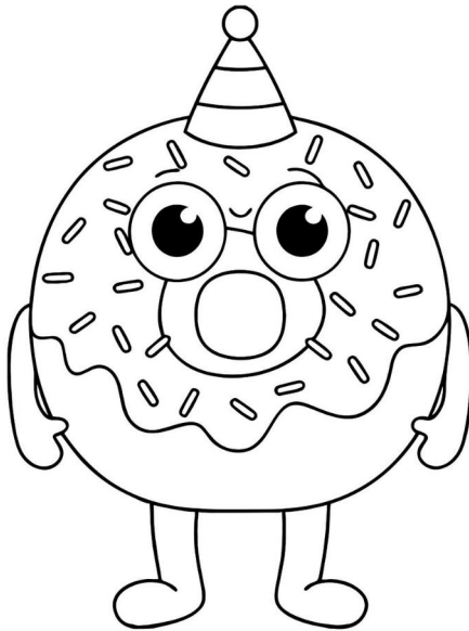
Torus Monster
